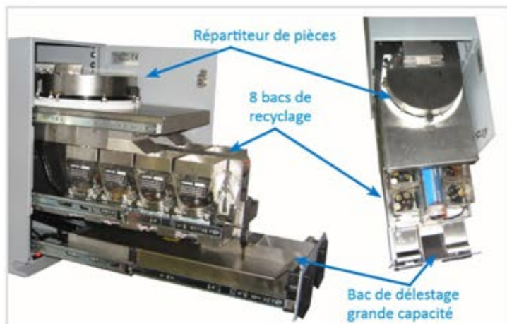
Module Pièces, ouverture à l'arrière
