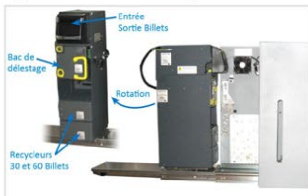
Module Billets, ouverture à l'arrière
